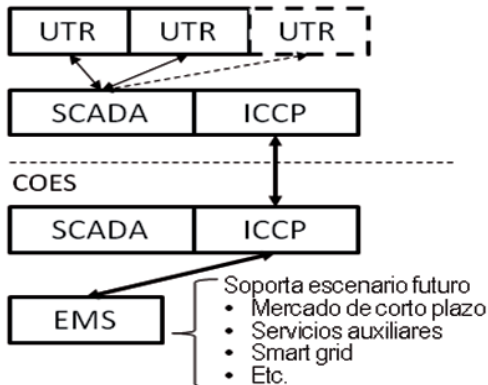
Figura 1.- flujo de datos desde las UTR (unidad terminal remota) en las subestaciones, los sistemas SCADA en los centros de control, la integración de los servidores ICCP, la integración con el EMS ( Energy Management System ) del COES a través de protocolo ICCP y como a partir de la operación del EMS se lograría nueva funcionalidad en beneficio de la operación y el mercado eléctrico.
