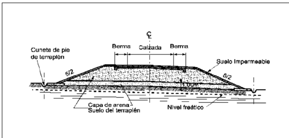
Figura N° 39: Protección del terraplén.
